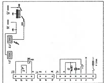
TYPE TM12F
