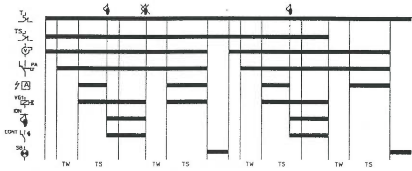
TYPE TM32F
