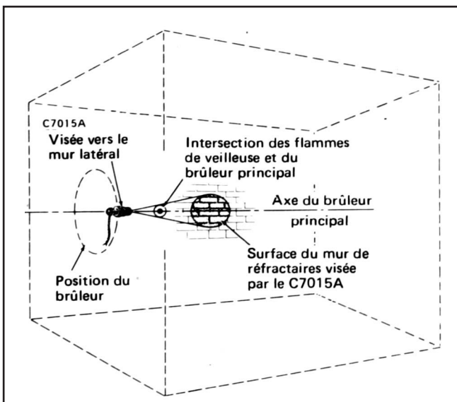
Fig. 4 — Détecteur infra rouge dirigé sur le mur latéral de la chambre de combustion. Fig. 7
