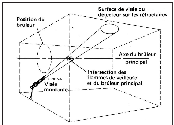
Fig. 5 -- Détecteur infrarouge dirigé sur un point situé en haut des réfractaires.
