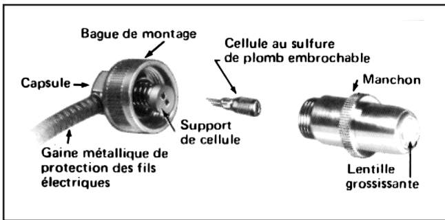
Fig. 8. Installation d'une cellule au sulfure de plomb
