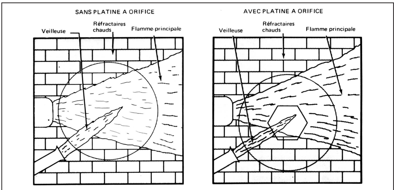
Fig. 3. Utilisation d'une platine à orifice pour réduire la surface de visée du détecteur sur l'intersection de la veilleuse et de la flamme du brûleur principal, ou sur une petite surface des réfractaires chauds.
