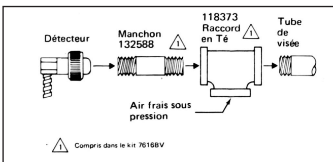
Fig. 7. Refroidissement par air sous pression
