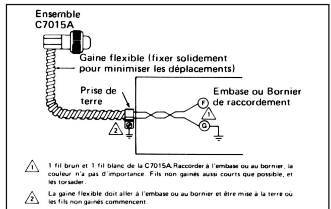
Fig. 10 - Câblage type d'une C7015A proche de la base de câblage ou du bornier
