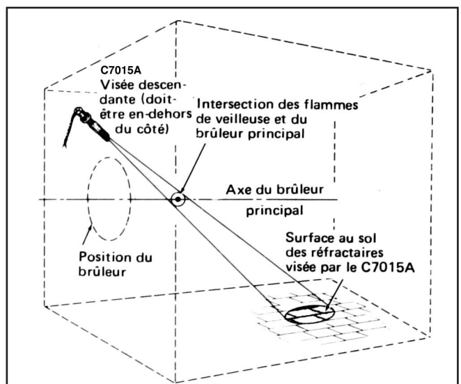
Fig. 6— Détecteur infrarouge dirigé sur le plancher de la chambre de combustion.
