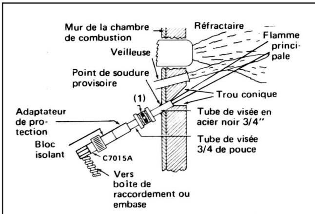
Fig. 9. Montage du détecteur à infrarouge C7015 (et accessoires)
