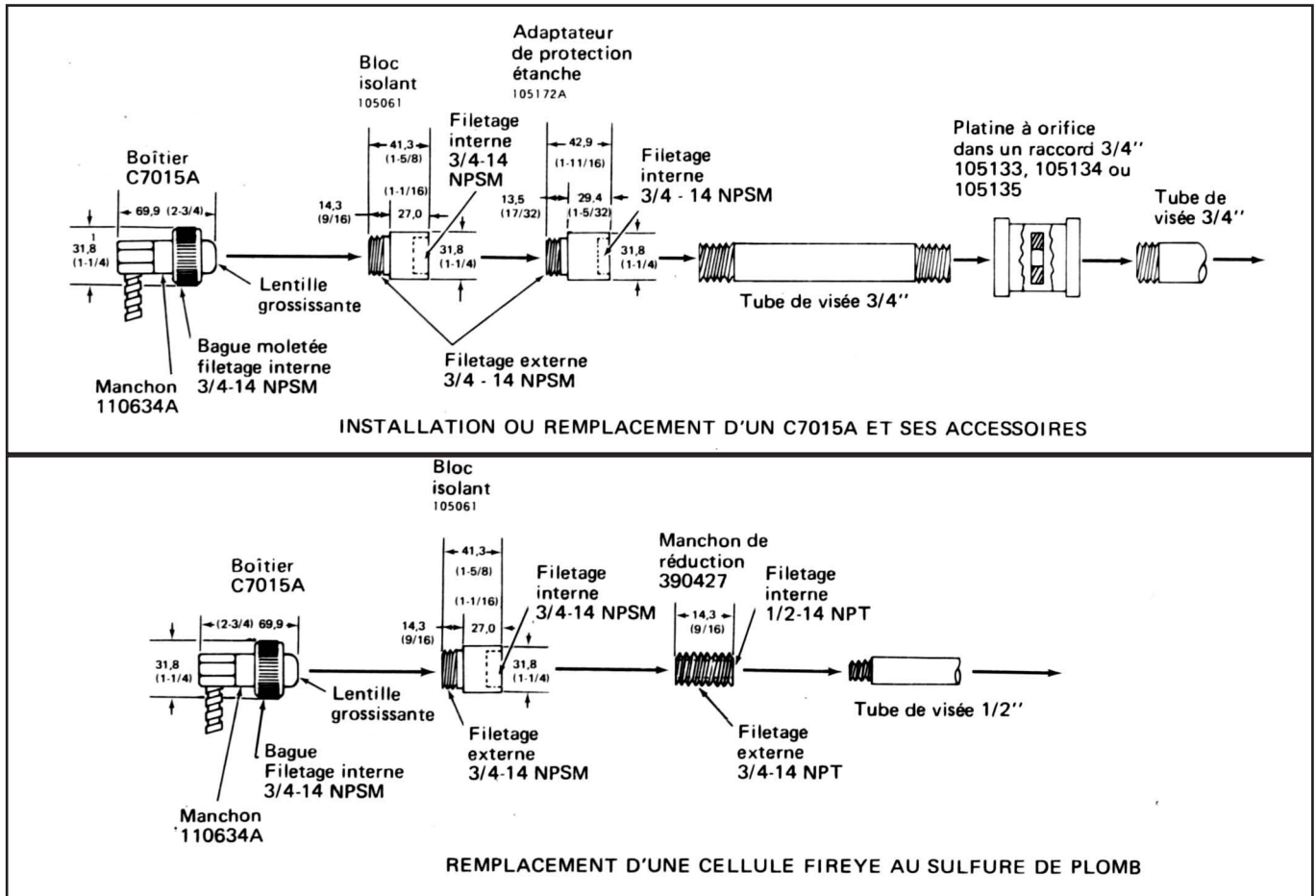
Fig. 1 Dimensions de montage d'une cellule C7015A et ses accessoires en millimètres (Inches entre parenthèses)
