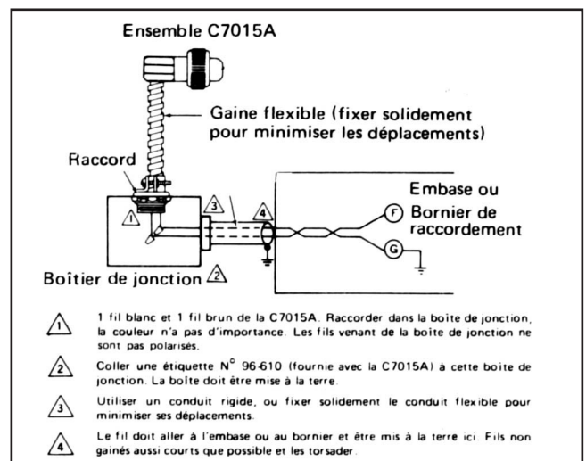
Fig. 11 - Câblage d'une C7015A éloignée de la base de câblage ou du bornier
