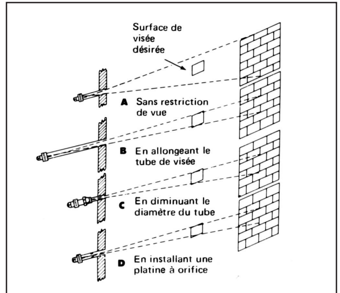
Fig. 2 Méthodes de réduction du champ de visée du détecteur.
