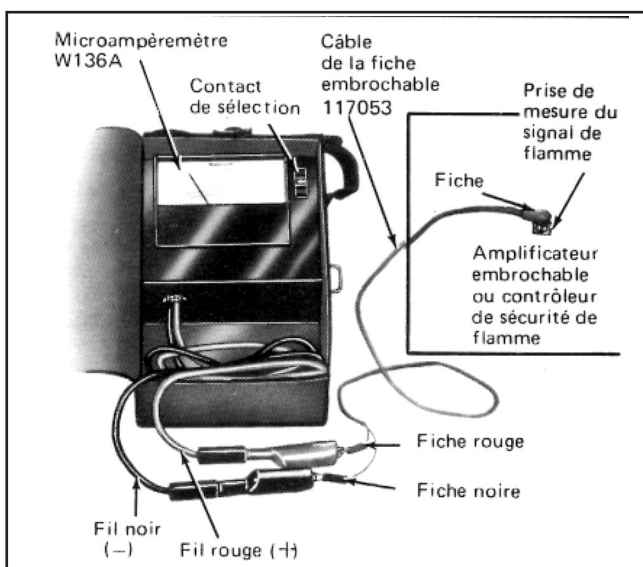
Fig. 12 - Mesure du signal de flamme
