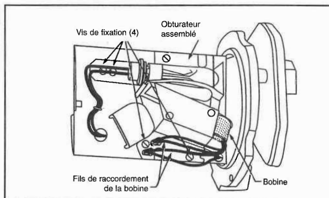
Figure 13 - Remplacement de l'ensemble bobine et obturateur sur la C7061A.
