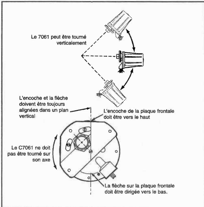
Figure 5 - Position de montage recommandée
