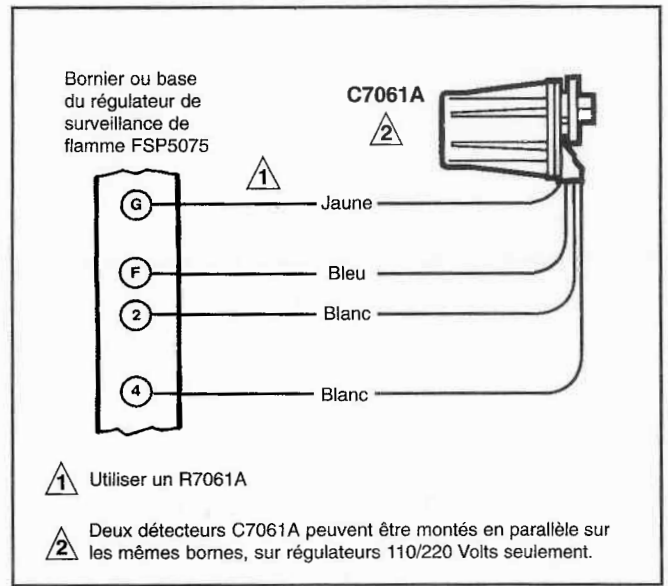
Figure 10.1 - Schéma de raccordement d'un C7061A avec un régulateur de surveillance de flamme FSP5075
