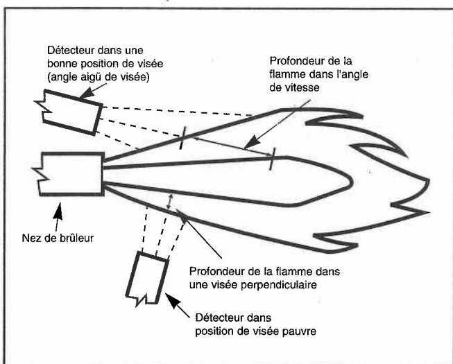
Figure 2 - Angle de visée du détecteur
