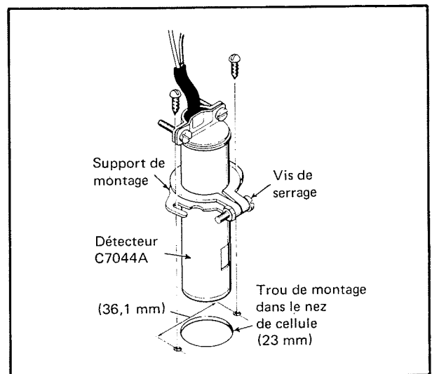
Fig. 7 — Montage de la C7044A sur un nez de brûleur
