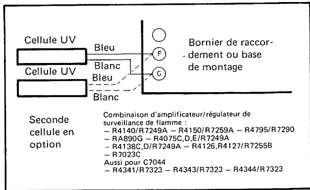
Fig. 8 — Schéma de câblage des cellules C7027A, C7035A et C7044A
