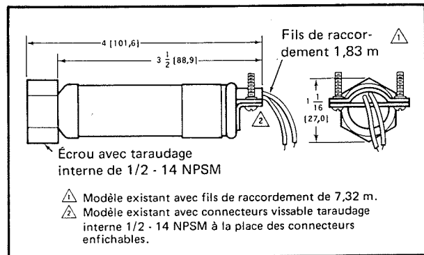
Fig. 1 — Dimensions d'installation de la cellule C7027A en mm
