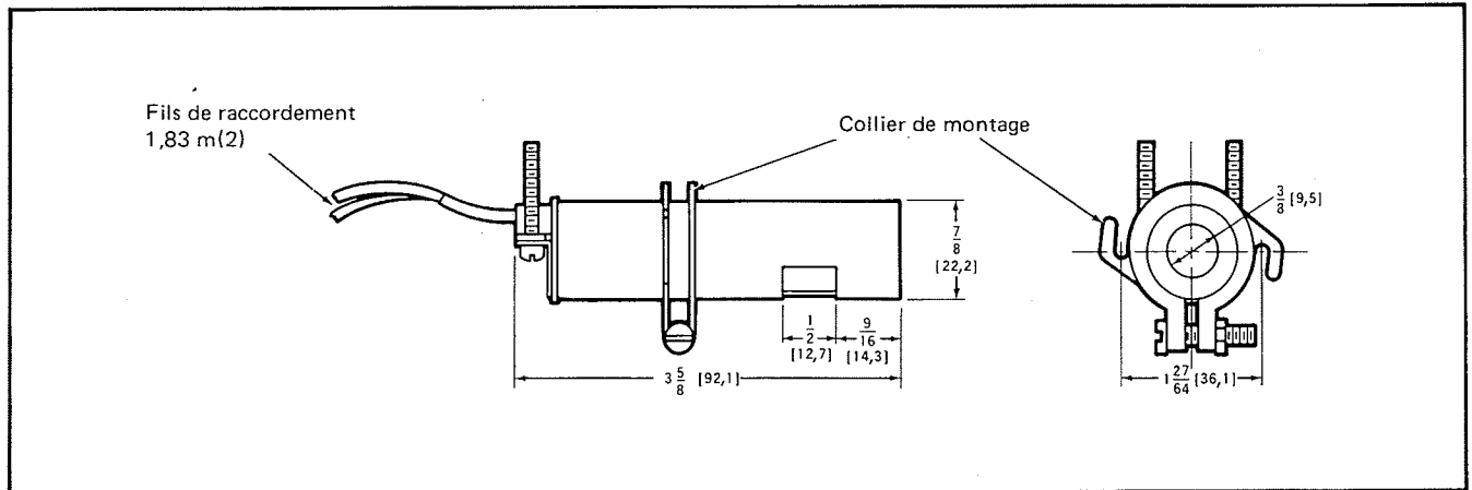
Fig. 3 — Dimensions d'installation de la cellule C7044A
