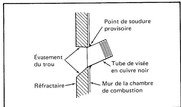
Fig. 4 — Montage du tube de visée
