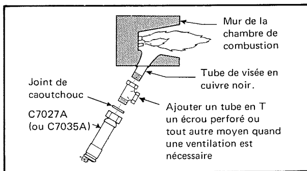
Fig. 6 — Montage de la cellule C7027A sur la chambre de combustion (vue de dessus). Le montage de la C7035A est similaire.
