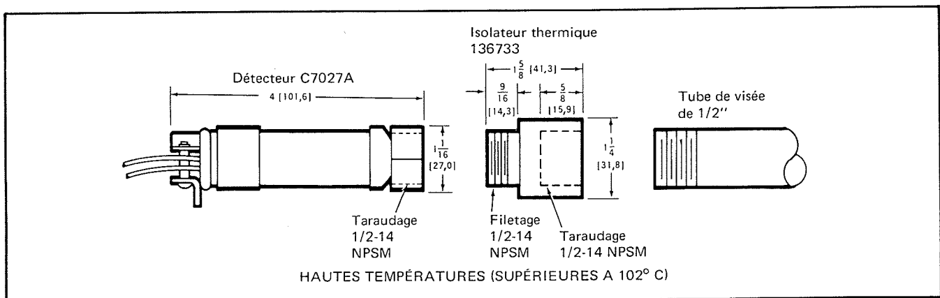
Fig. 5 — Dimensions de montage de l'isolateur thermique 136733
