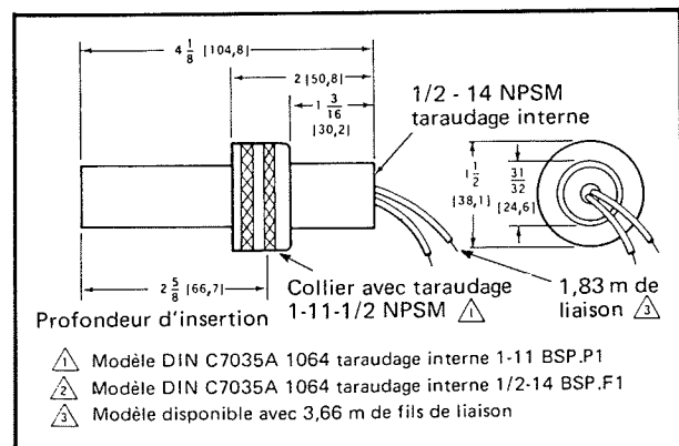
Fig. 2 — Dimensions d'installation de la cellule C7035A en mm
