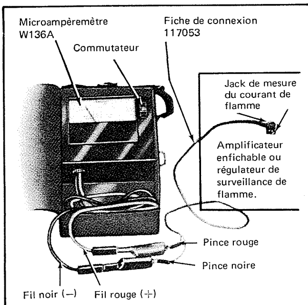
Fig. 9 — Mesure du courant de flamme
