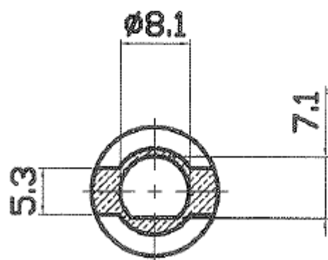
SEZ. A-A
