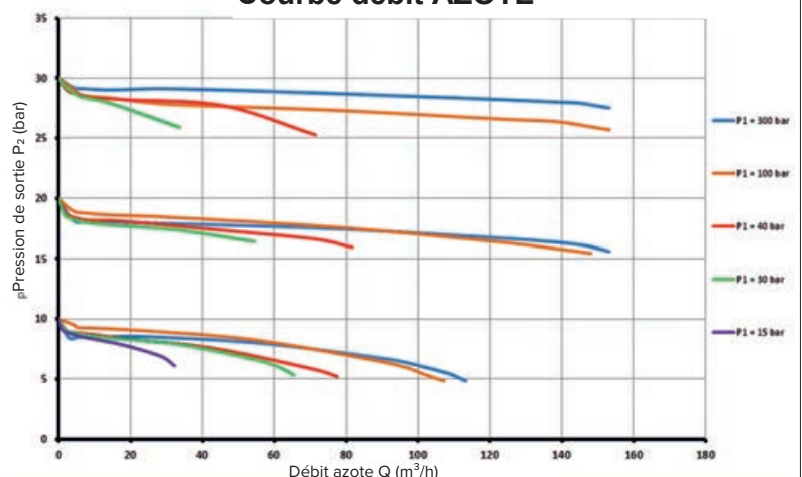
Courbe débit AZOTE
